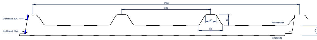
FALK Dach 80
